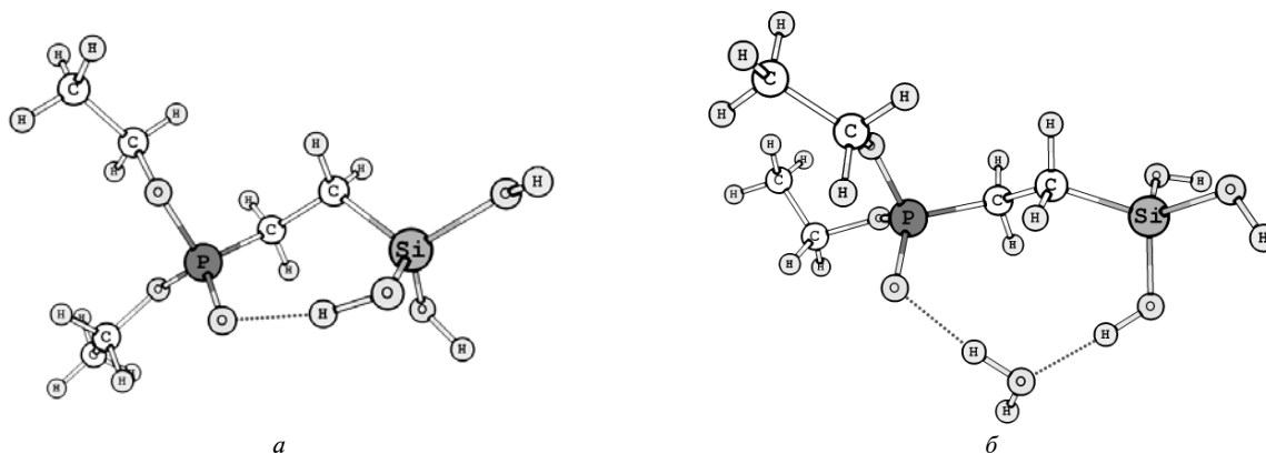
Рис. 2. Оптимізована геометрія фрагментів (\text{HO})_2\text{Si}(\text{OH})(\text{CH}_2)_2\text{P}(\text{O})(\text{OC}_2\text{H}_5)_2 , що містять водневий зв'язок: а – без участі води; б – за участю молекули води
