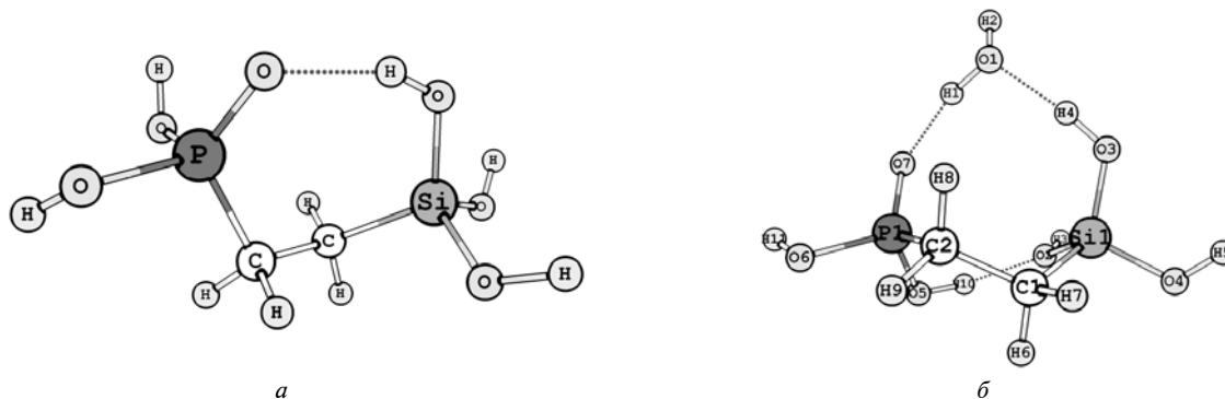
Рис. 3. Оптимізована геометрія фрагментів (\text{HO})_2\text{Si}(\text{OH})(\text{CH}_2)_2\text{P}(\text{O})(\text{OH})_2 , що містять водневий зв'язок: а – без участі води; б – за участю молекули води
