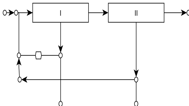
Рис.2. Схема двухступенчатой ОО установки с рециклом части концентрата (редактор yEd)
