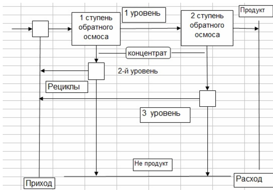
Рис. 1. Схема двухступенчатой ОО установки с рециклом части концентрата (редактор Excel)
